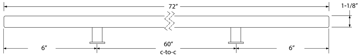
72" Square Door Pull 86188
