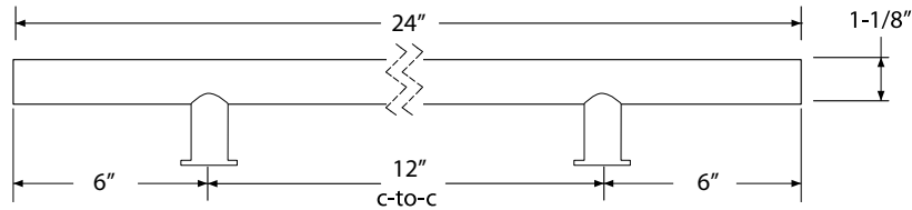
24" Round Door Pull 86193
